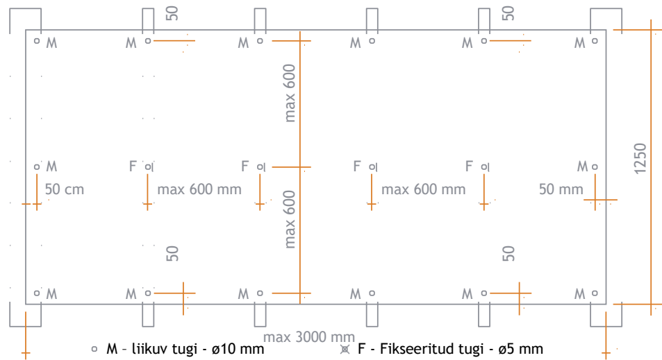
Paneeli kinnituskohad
